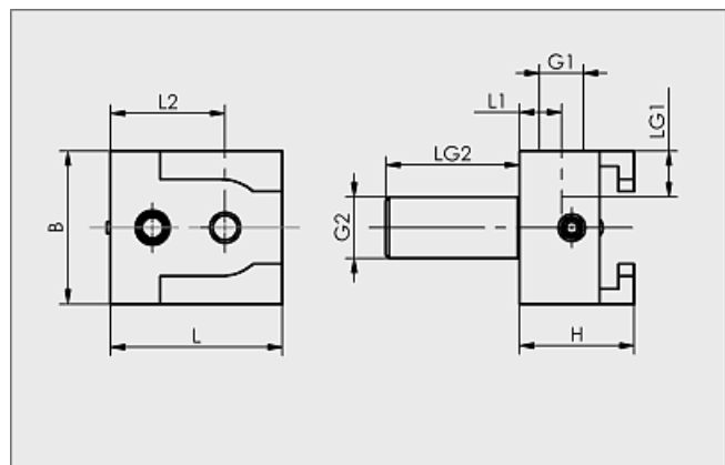
Suction-pad holder HTR-S G2 RA
