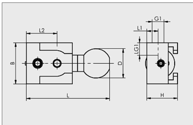
Suction-pad holder HTR-S A3 RA
